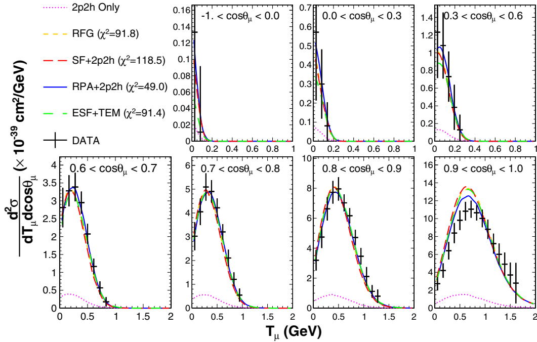
(b) Antineutrino
